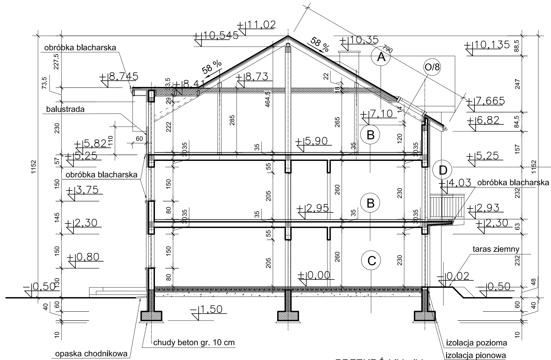
PRZEKRÓJ IV - IV
